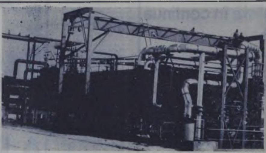
Vedere generală a instalațiilor Uzinei experimentale pentru desalinizarea apei de mare la Nuakshott (Mauritania), prima de acest fel din Africa de vest.
