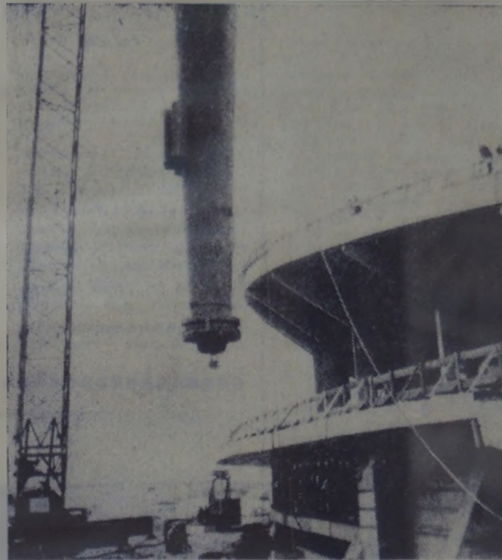
R.F.G. Zilele acestea au început lucrările acoperisului care se va întinde pe circa 250.000 de m.p. al terenului olimpic de la München, acoperind bazinul de înot, stadionul, etc. Montat pe piloni de oțel înalți, ajungînd pînă la aproximativ 80-90 m au în interior scări pe care să poată circula muncitorii. În foto: Așezarea unui din pilonii de oțel cu ajutorul unei macarale de 500 tone
